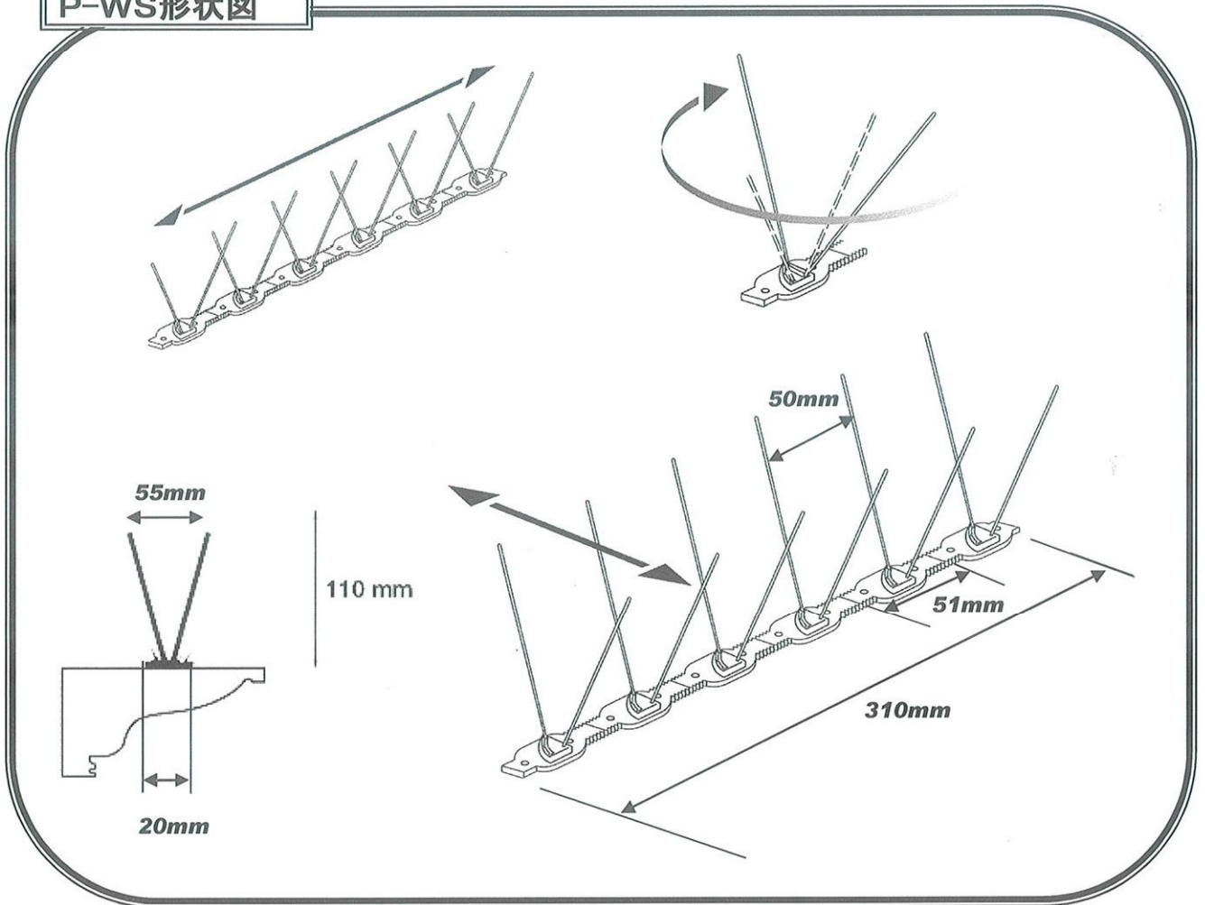
P-WS形状図
